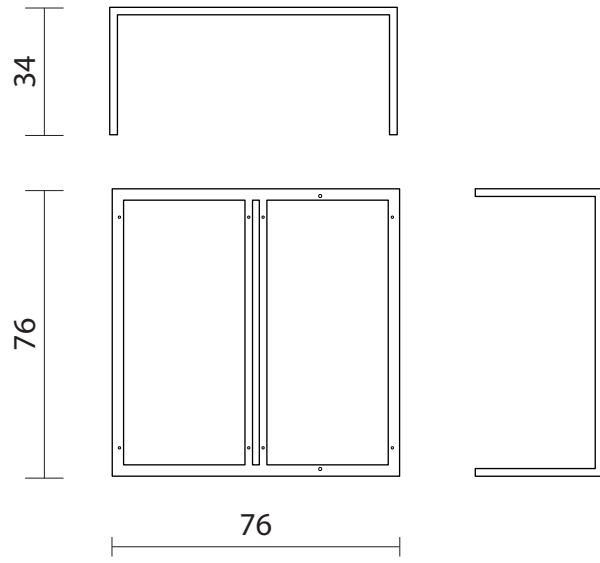
Double frame (SBTH01-NE)
